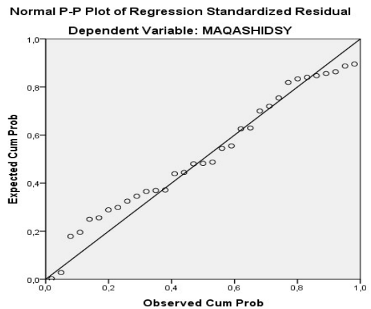
Sumber : Output SPSS yang diolah Gambar 2. Hasil Uji Normalitas Dengan Grafik Normal Plot
