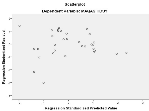
Sumber : Output SPSS yang diolah Gambar 1. Hasil Uji Heterokedastiitas Dengan Scatterplot
